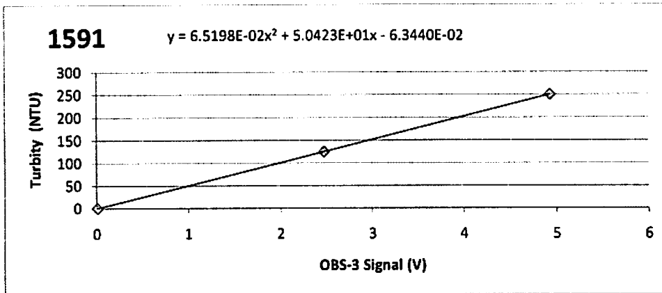
Volt Calibration
