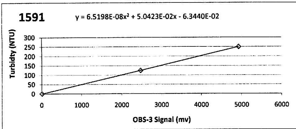
Volt Calibration
