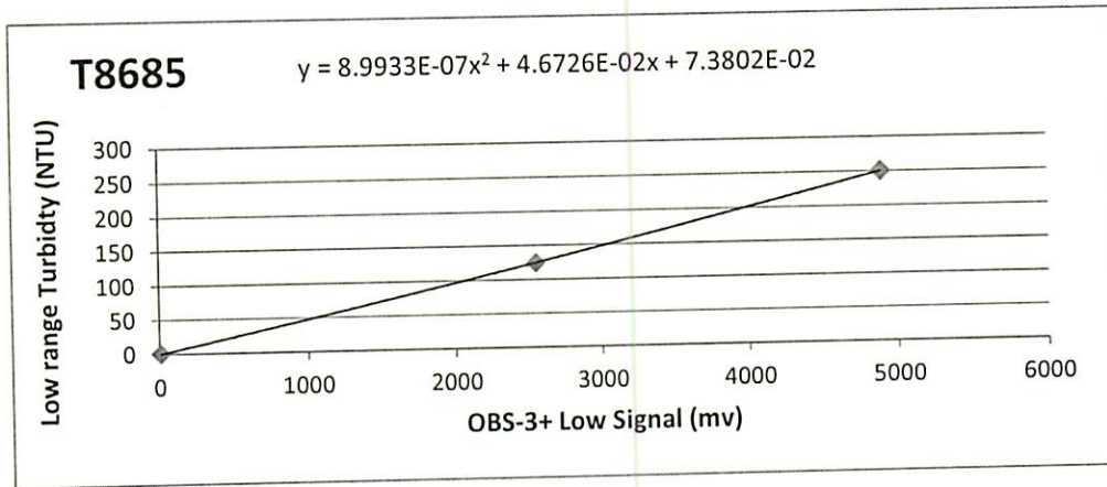
Milli-Volt Calibration
